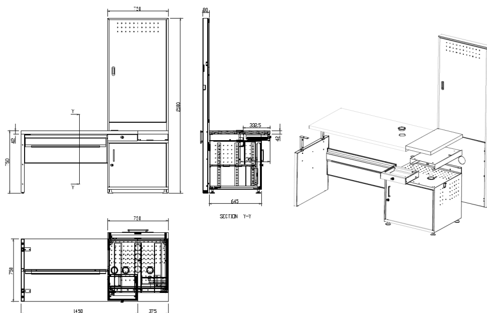
Figura 4 – Posto Individual – Medidas gerais e Perspetiva de componentes
