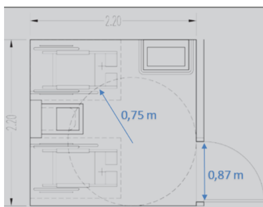
Figura 2 – Exemplo de configuração das Instalações Sanitárias
