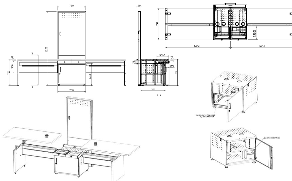
Figura 5 – Posto Duplo – Medidas gerais e Perspetiva de componentes
